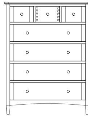
3 + 4 CHEST H: 1165 W: 900 D: 450
