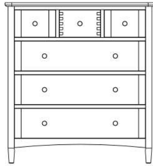
3 + 3 CHEST H: 965 W: 900 D: 450
